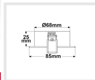
113713 | Einbaurahmen rund, Lochausschnitt 68mm, Alu Nickel-Satin, für
