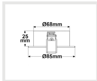
115694 | Einbaurahmen rund, Lochausschnitt 68mm, Alu gebürstet, für
