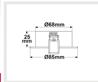
115695 | Einbaurahmen eckig, Lochausschnitt 68mm, weiß, für GU10/MR16 Spots
