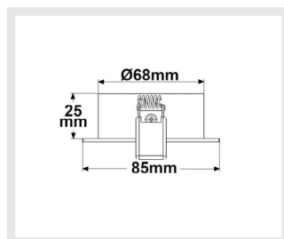
113712 | Einbaurahmen rund, Lochausschnitt 68mm, Alu weiß, für GU10/MR16
