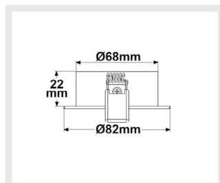
113712 | Einbaurahmen rund, Lochausschnitt 68mm, Alu weiß, für GU10/MR16
