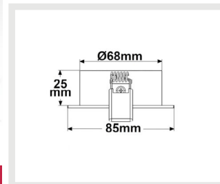
115697 | Einbaurahmen eckig, Lochausschnitt 68mm, Alu gebürstet, für
