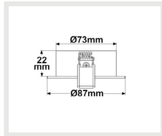
114986 | Einbaurahmen Ion rund, Lochausschnitt 73mm, chrom, für GU10/MR16 Spots
