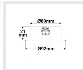
114005 | Einbaurahmen rund, Lochausschnitt 80mm, schwarz + schwarz-gold, für
