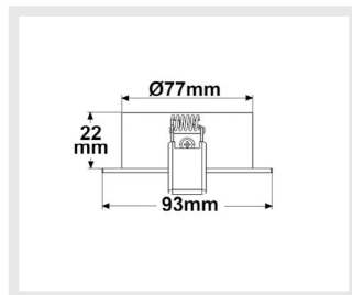
111062 | Einbaurahmen BRUSH eckig, Lochausschnitt 78mm, Alu gebürstet, für
