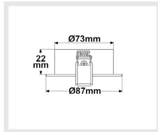
111048 | Einbaurahmen rund, Lochausschnitt 73mm, nickel satin, für GU10/MR16
