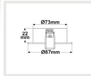
111047 | Einbaurahmen rund, Lochausschnitt 73mm, weiß, für GU10/MR16 Spots
