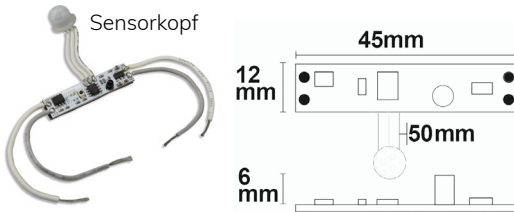
113726 LED Mini-Switch PIR Bewegungssensor für Profile, max. 24V/5A
