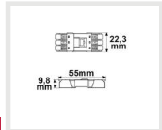
116148 | Anschlussklemme 2x2-polig, 0,5-2,5mm 2 , max. 450V/16A
