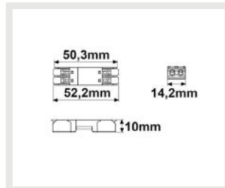
116147 |* Durchgangs-Steckverbinder 2-polig Input, 2x2-polig
