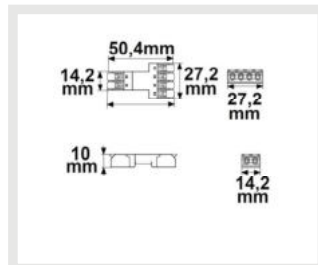
116149 | Anschlussklemme 2x3-polig, 0,5-2,5mm 2 , max. 450V/16A
